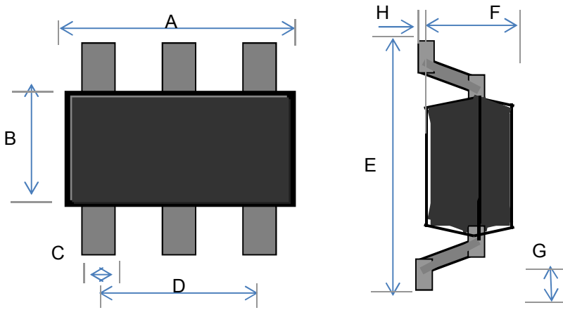
SOT-363
