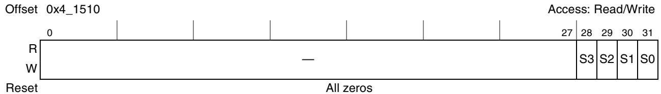
Figure 10-29. Message Status Register (MSR)
