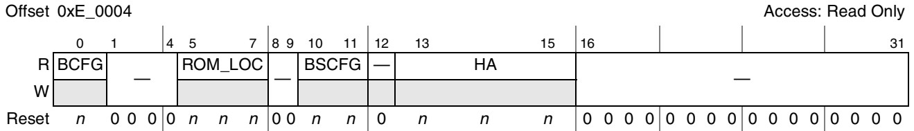
Figure 20-2. POR Boot Mode Status Register (PORBMSR)
