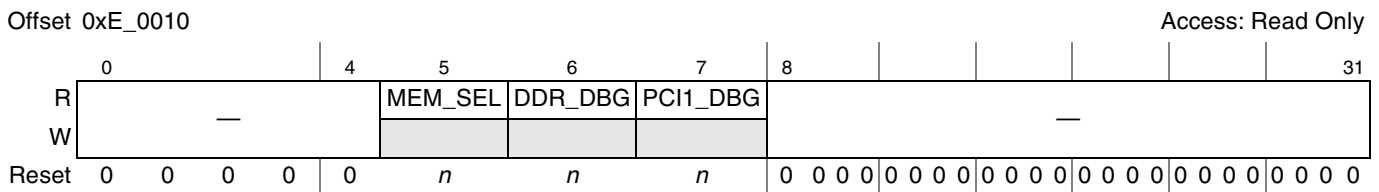
Figure 20-5. POR Debug Mode Status Register (PORDBGMSR)
