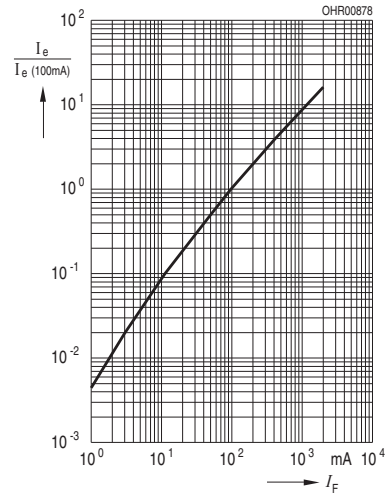
Radiant Intensity 2) page 13 Strahlstärke 2) Seite 13 I_e / I_e(100 \text{ mA}) = f(I_F) , single pulse, t_p = 25 \mu\text{s} , T_A = 25^\circ\text{C}
